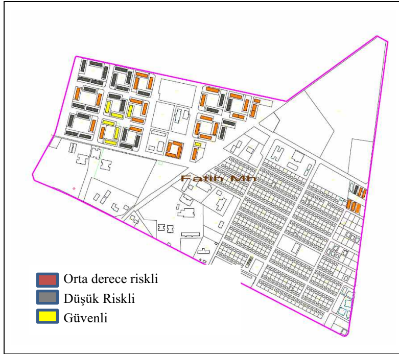
Şekil 9. Binaların risk durumuna göre bölgesel dağılımları
