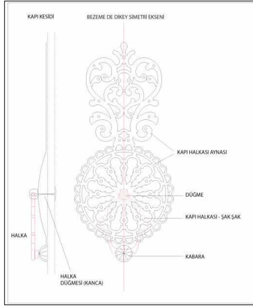
Çizim 6. Kemaliye kapılarında halka ve halka (şakşak) aynasındaki bölümler.
