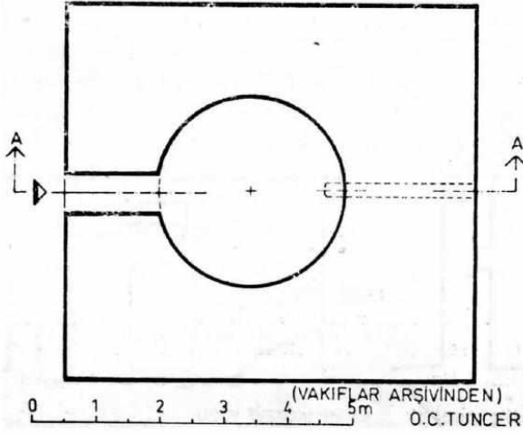
Çizim 11. Midilli Baba türbesi planı (O.C.Tuncer'den)
