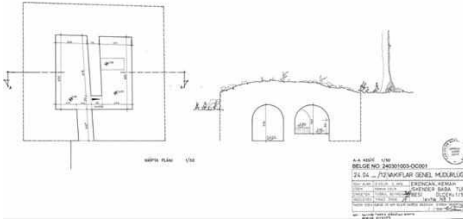
Çizim 10. İskender Baba Türbesi plan ve kesiti
