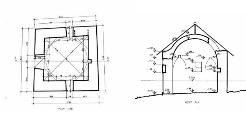
Çizim 8. Ali Baba Türbesi planı Çizim 9. Ali Baba Türbesi kesit
