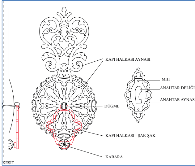
Çizim 3. Kemaliye kapı halkasına ve kilit aynasına ait birer örnek.
