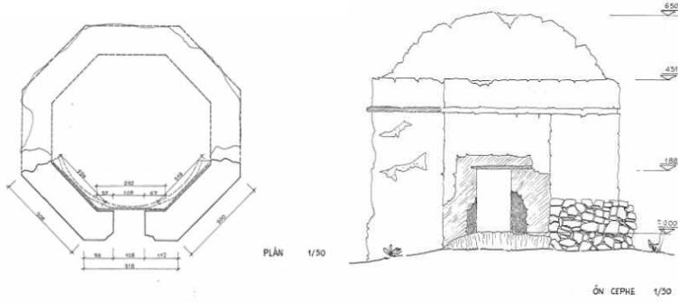
Çizim 4. Anonim Kümbet planı Çizim 5. Anonim Kümbet, kesit
