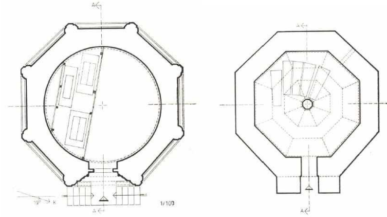
Çizim 1. Melik Gazi Kümbeti, cenazelik planı (O. C. Tuncer'den)
