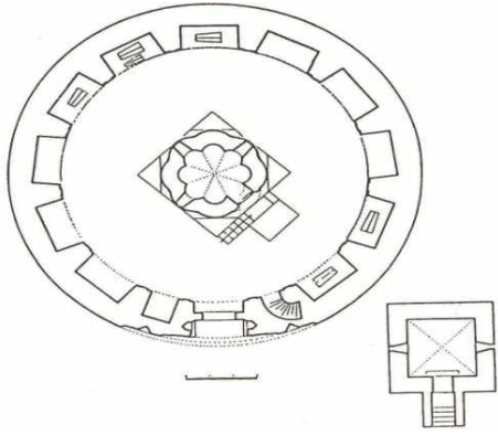
Çizim 12. Tercan Mama Hatun Kümbeti planı (S.K.Yetkin'den)
