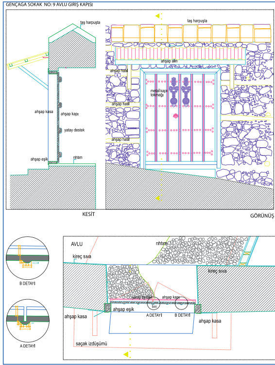
Çizim 1. Kemaliye Evi Kanatlı Kapı Kesit, Plan, Görünüş 31
