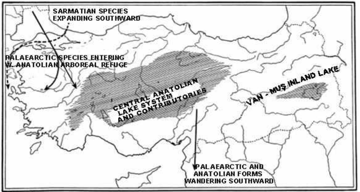
Şekil 3. Buzul önemi boyunca Anadolu faunasının hareketleri (Koswig, 1955).
