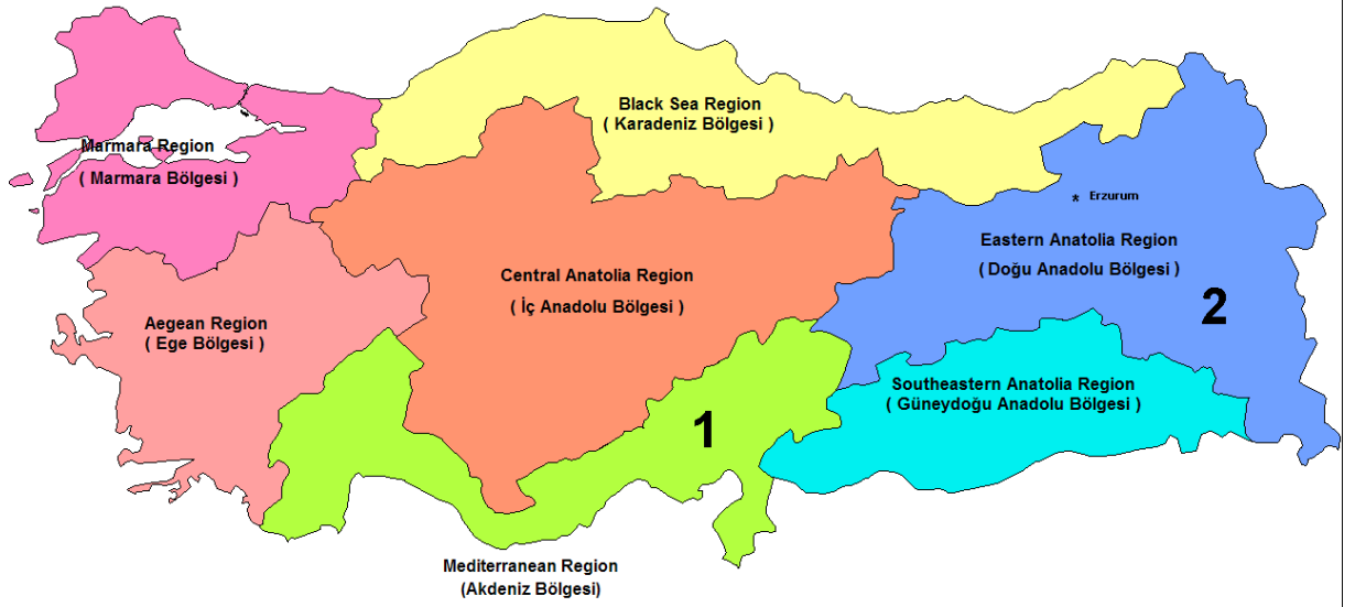
Şekil 5. Yedi coğrafik bölgenin endemizm durumu (İncekara, 2012).
