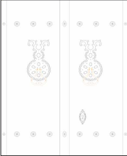
Çizim 14. Dört yolağı Mah. Cumhuriyet Cad. 84 No'lu ev, Ali Güven Evi (Kasapgil'in Ev) kapısına ait bezemeli metal plakanın çizimi
