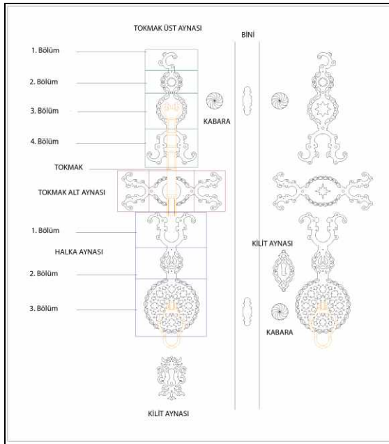
Çizim 4. Bezeme açısından Kemaliye kapı tak tokmağı ve tokmak aynası formlarına örnek.
