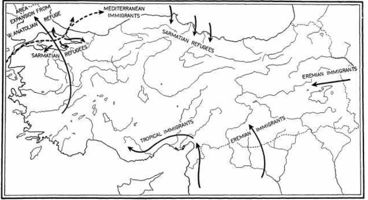
Şekil 4. Anadolu faunasının son buzul devri boyunca hareketleri (Koswig, 1955).
