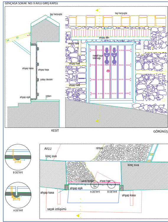
Çizim 1. Kemaliye Evi Kanathı Kapı Kesit, Plan, Görünüş 31
